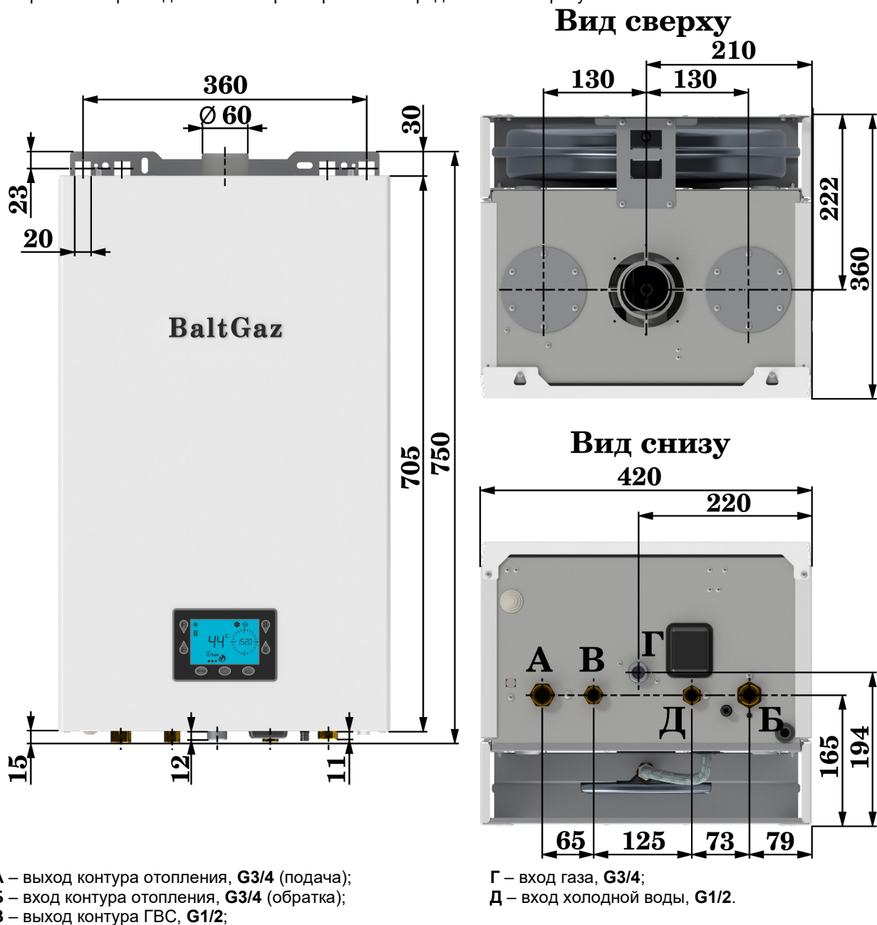
Рис. 1 Габаритные и присоединительные размеры котлов
